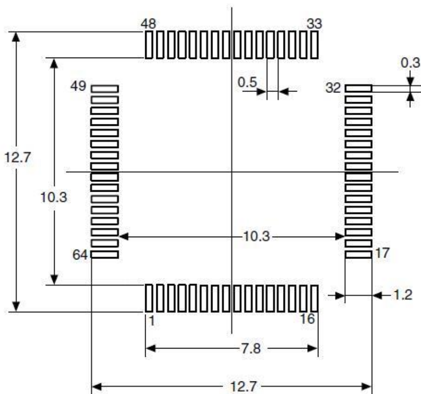
图 16 LQFP64-64 引脚, 10×10mm 焊接 Layout 建议
