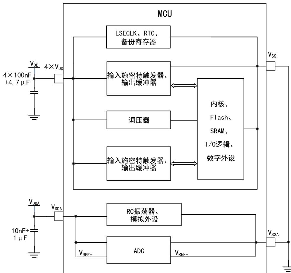
图 5 电源方案
