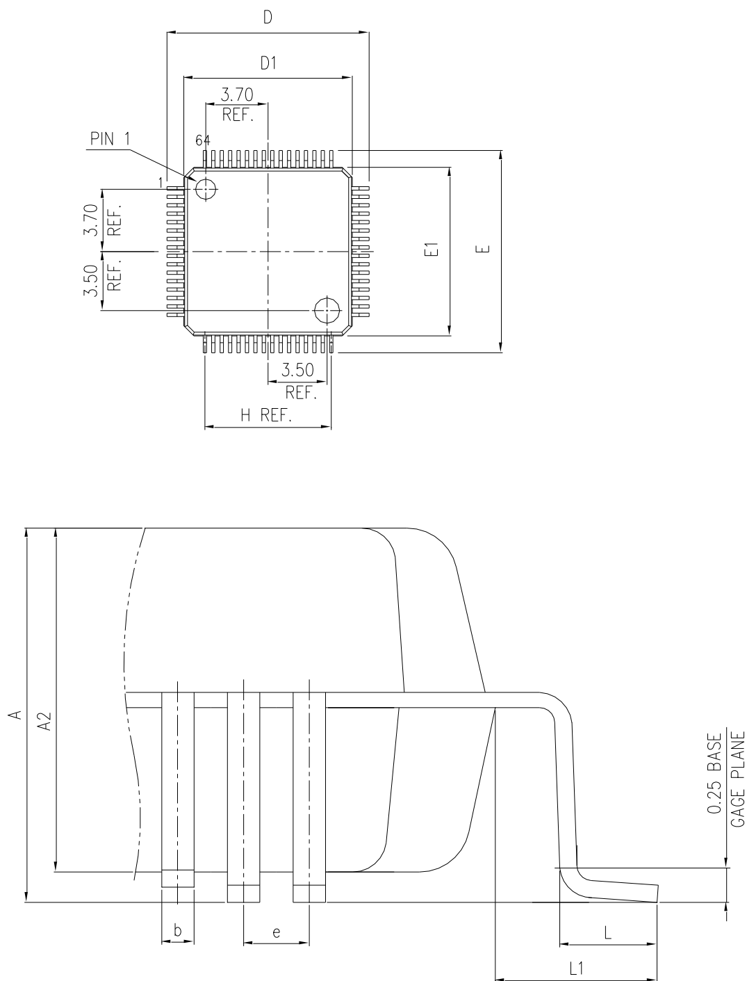
图 15 LQFP64 封装图
