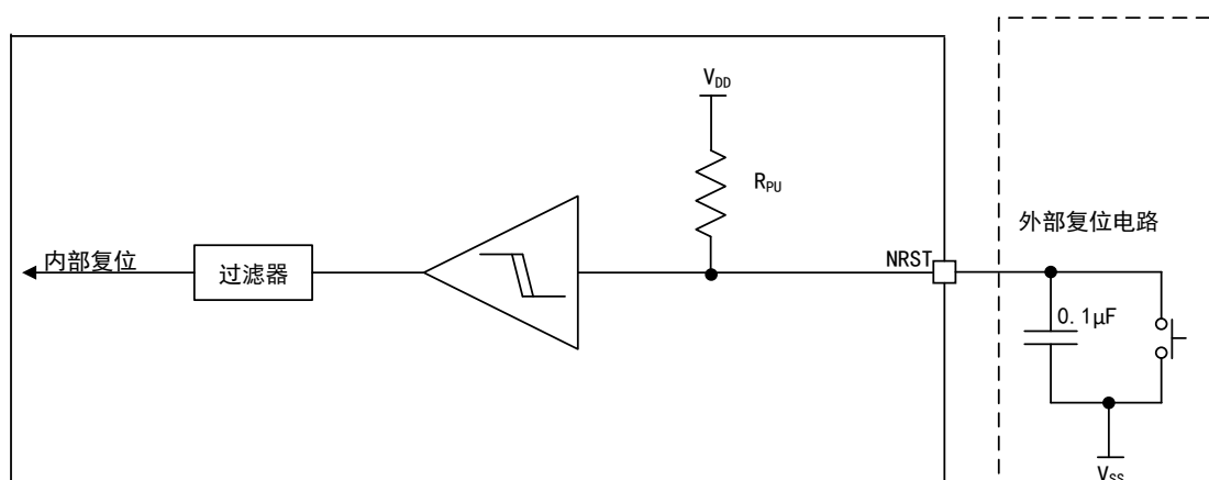
图 10 NRST 引脚保护推荐方案
