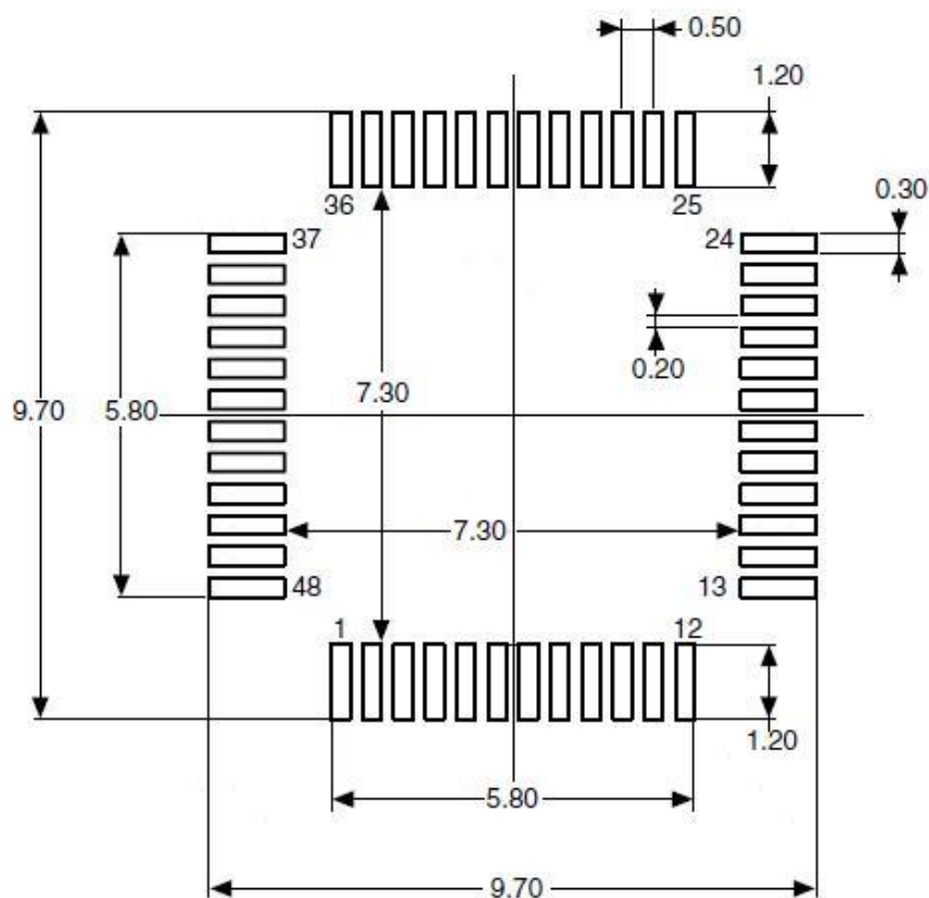
图 19 LQFP48, 7×7mm 焊接 Layout 建议
