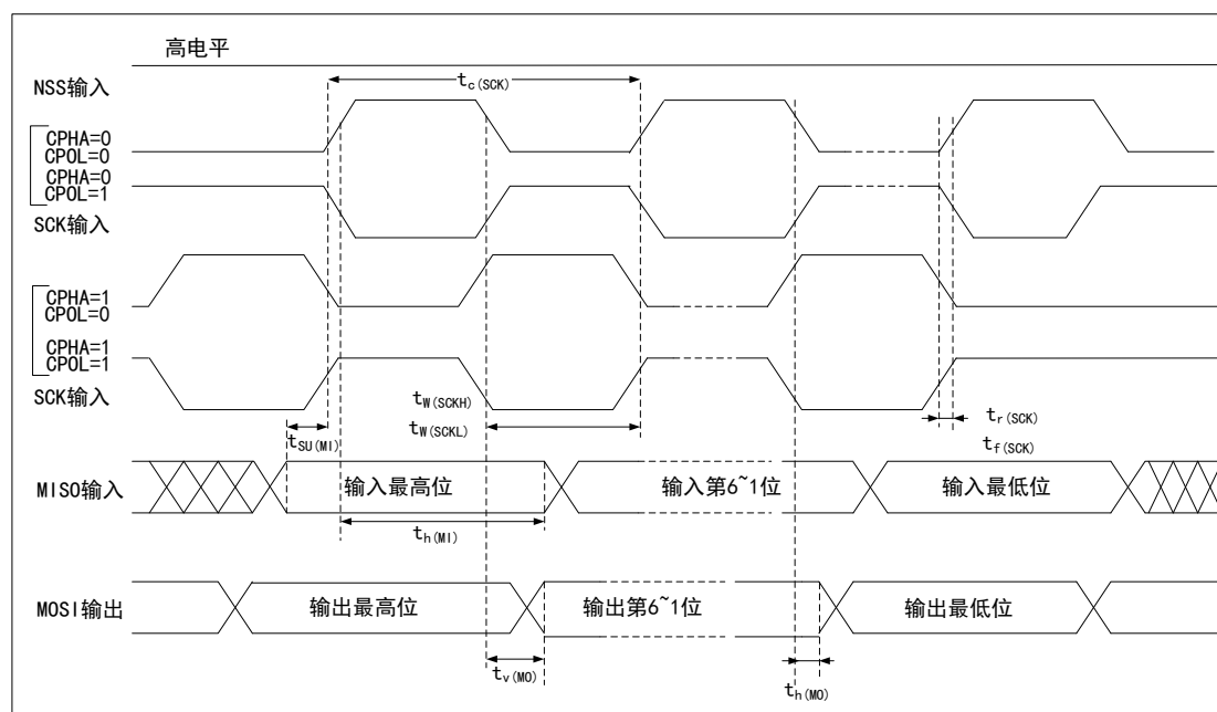
图 14 SPI 时序图—主模式
