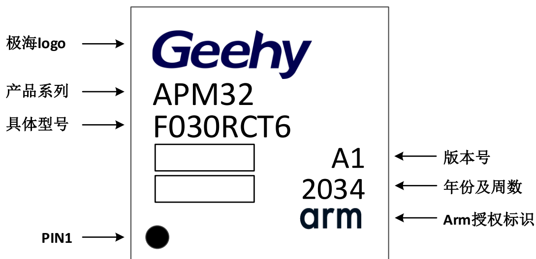
图 17 LQFP64-64 引脚，10×10mm 封装标识
